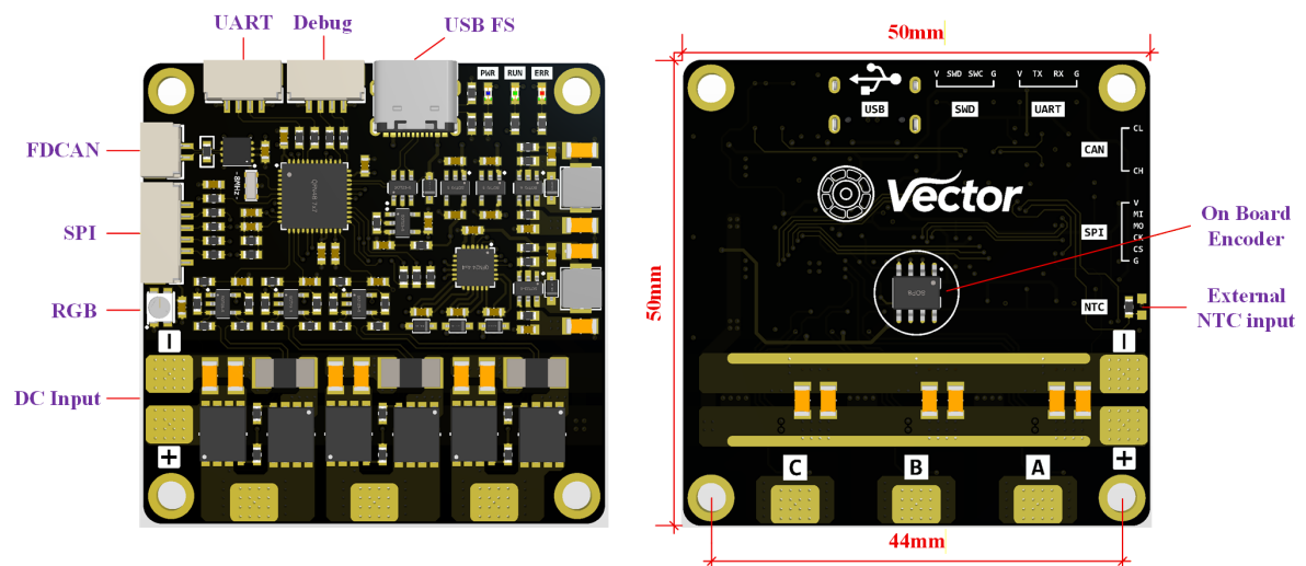
图2-1 驱动器布局示意图
